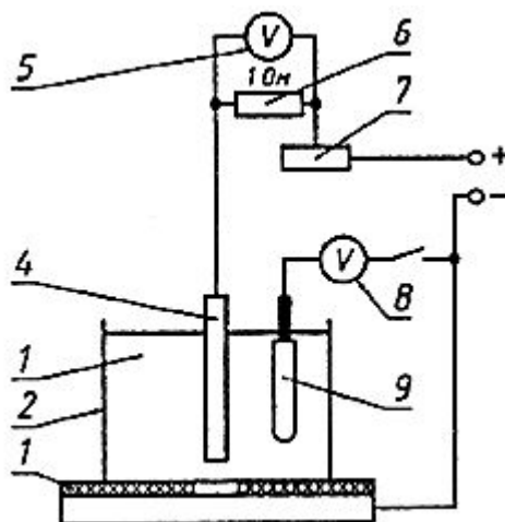
1 - пластина (карта) - испытуемый образец; 2 - труба из полиэтилена; 3 - электролит; 4 - инертный анод; 5 и 8 - вольтметры; 6 - эталонное сопротивление; 7 - реостат; 9 - электрод сравнения Рисунок В.4 - Схема проведения испытания образцов покрытий на пластинах (картах) для определения площади отслаивания с применением инертного анода
